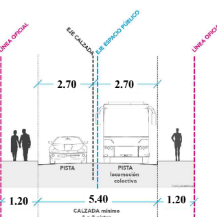
SECCION DE CALLES
